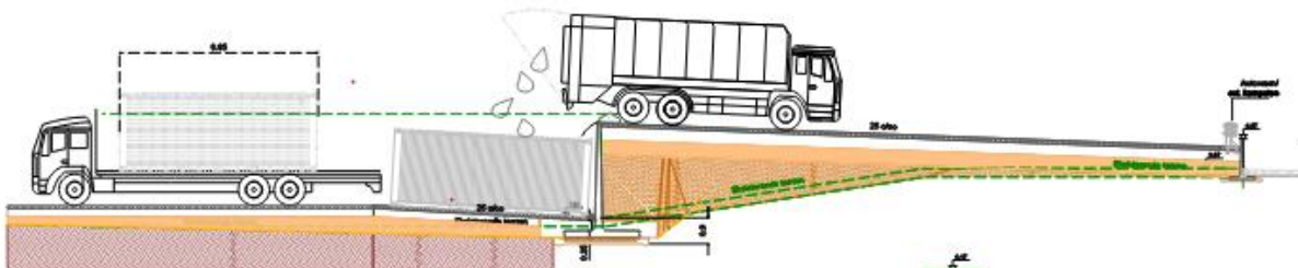
Princip for funktionalitet og udformning af ramper mv. på omlastepladsen.
